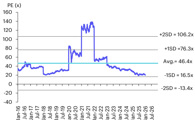
Figure 4: PE Band
