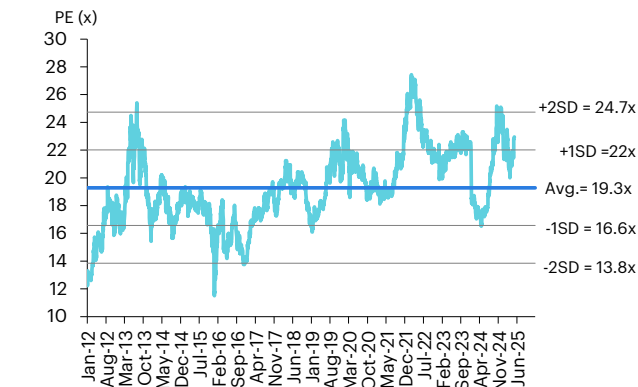
Figure 9: PE Band
